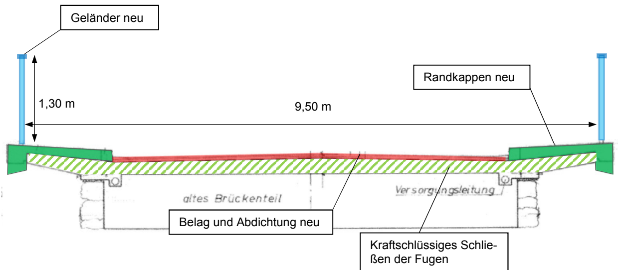
Querschnitt
