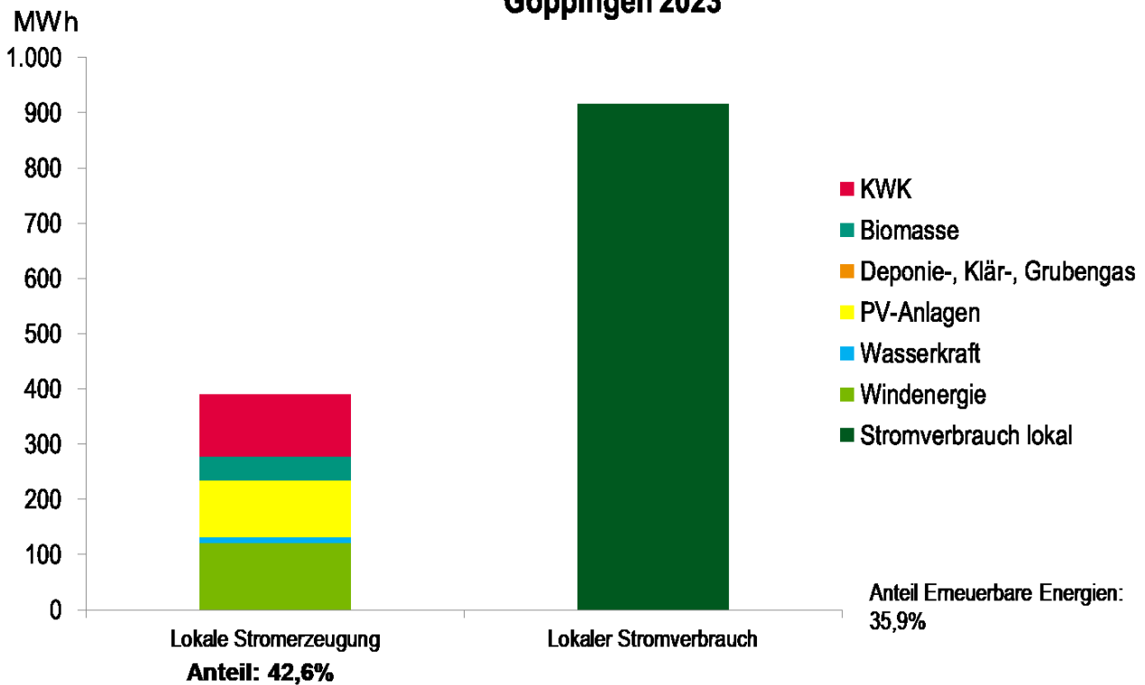
Abbildung 4: Stromerzeugung und Stromverbrauch im Landkreis Göppingen 2023
