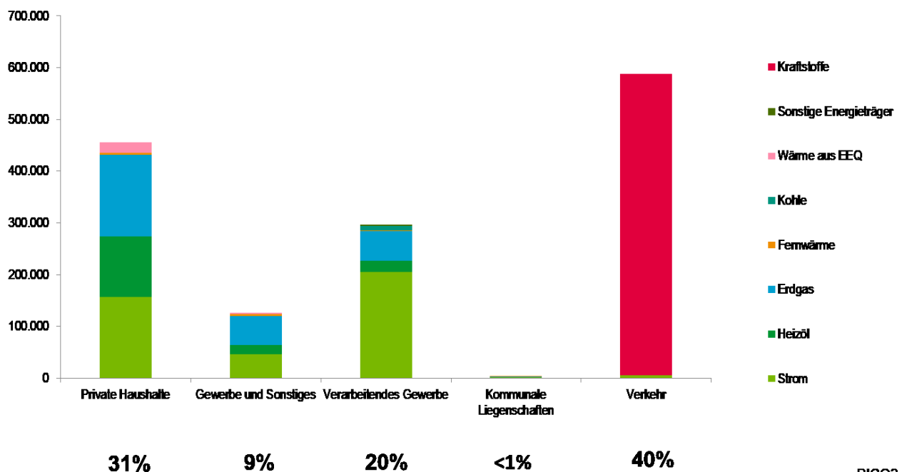
Abbildung 2: TGH-Emissionen nach Sektoren 2023
