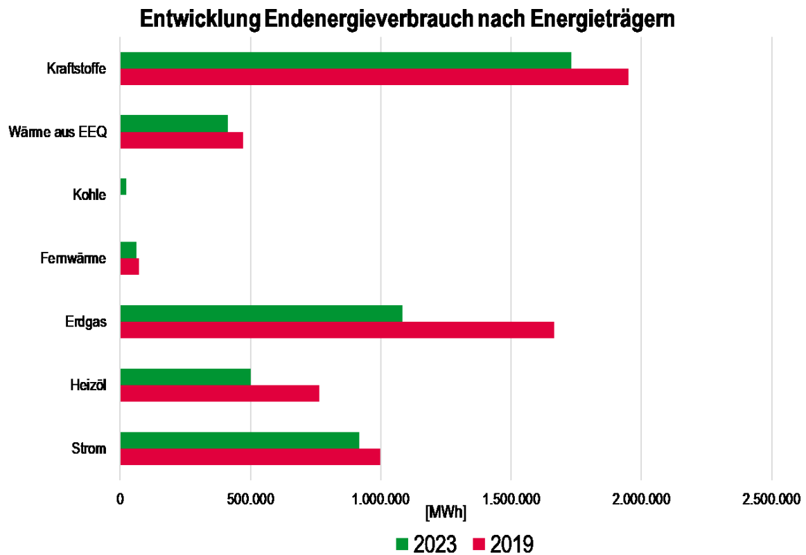
Abbildung 1: Entwicklung des Endenergieverbrauchs nach Energieträgern
